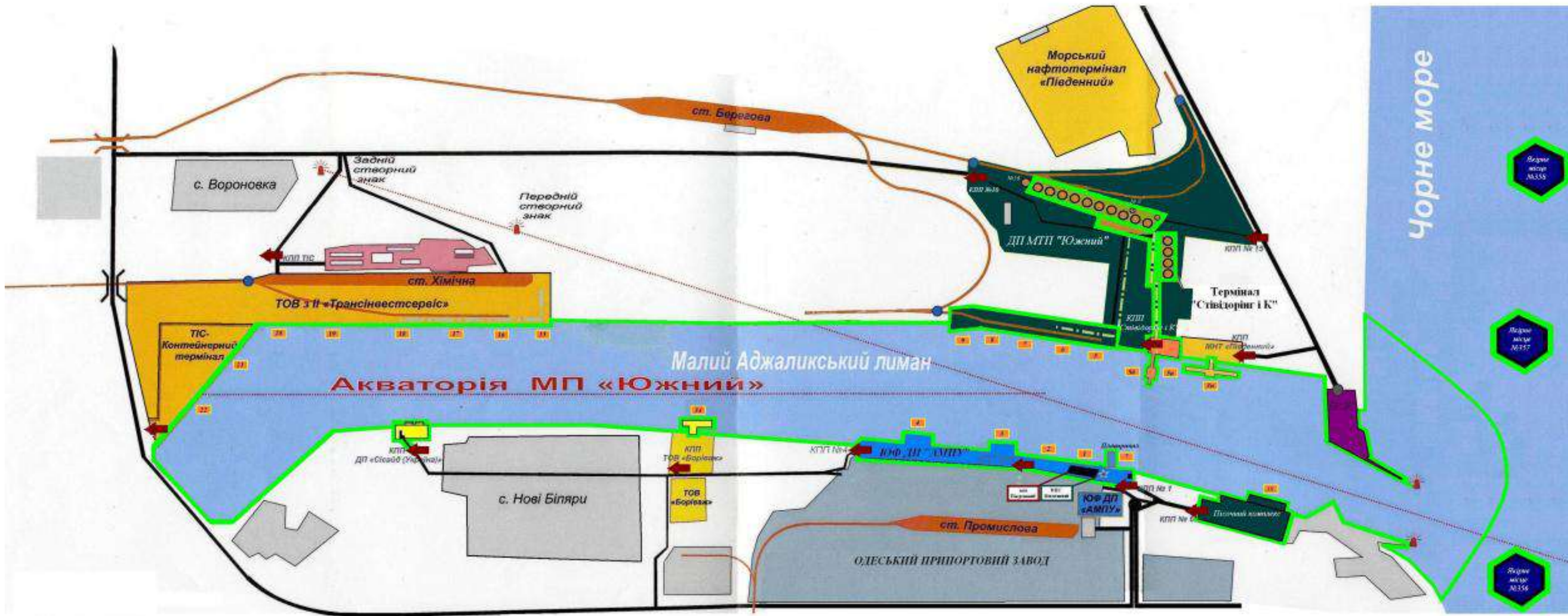
Схема території пункту пропуску для міжнародного морського вантажного сполучення "Морський торговельний порт "Южний"
